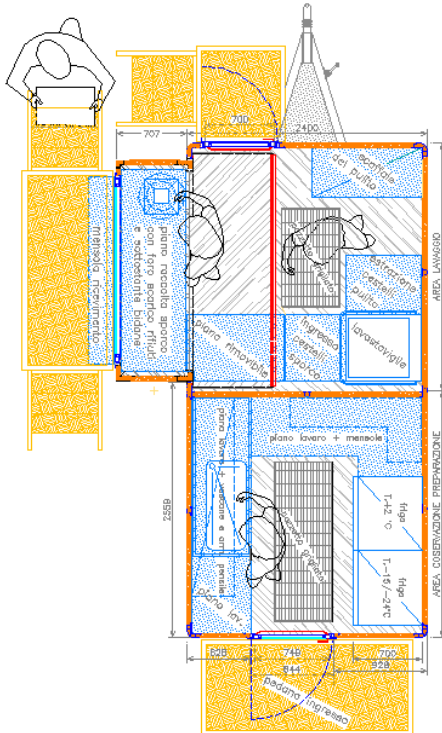
Vista/disegno in pianta del complessivo in operativo
