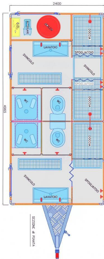
Ansicht/Planzeichnung des Ganzen
